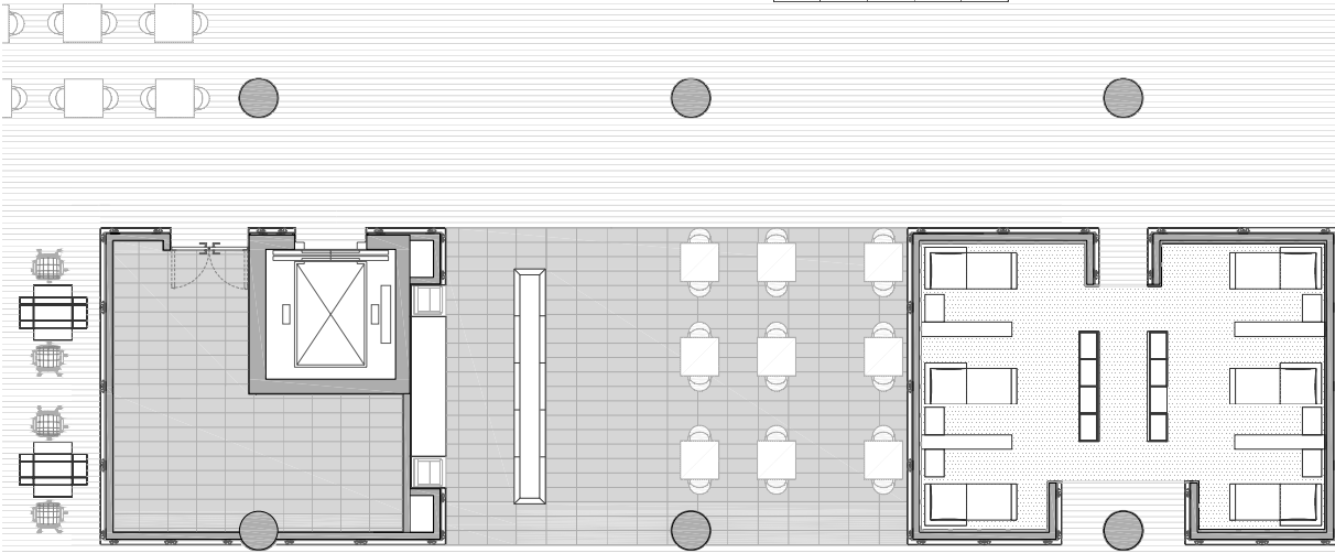
DETALLE DE UNA PARTE DE LA PLANTA
